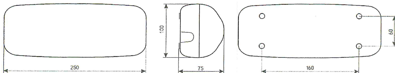
Рис. №2 Габаритный чертёж.
